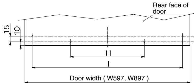
< Door sliding profile >
