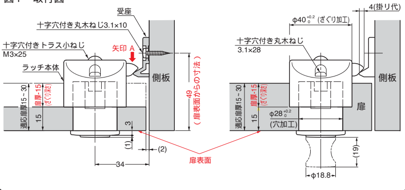
図1 取付図
